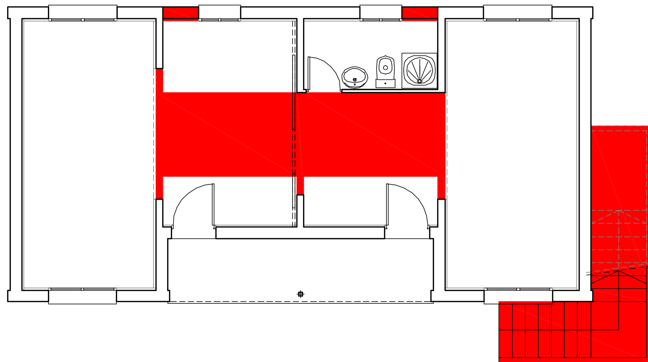
OBRA NOVA PLANTA BAIXA ESC. 1/50
